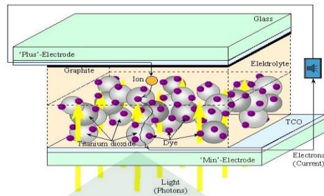
Gambar 2.2 Skema DSSC (Ekasari dan Yudhoyono, 2013: 16)
