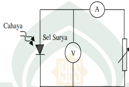
Gambar 4.3 Rangkaian pengukuran karakteristik I-V
