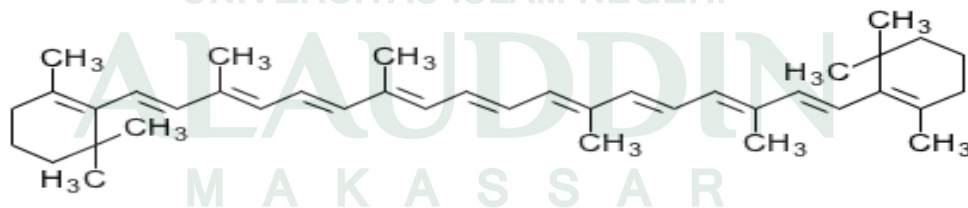
Gambar 2.6 \beta -karoten
