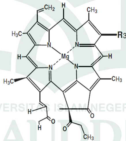
Gambar 2.8 Struktur Klorofil a
