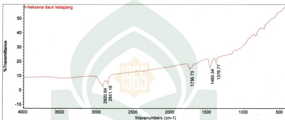
Gambar 4.4 Hasil Serapan IR Ekstrak Daun Ketapang n-heksan
