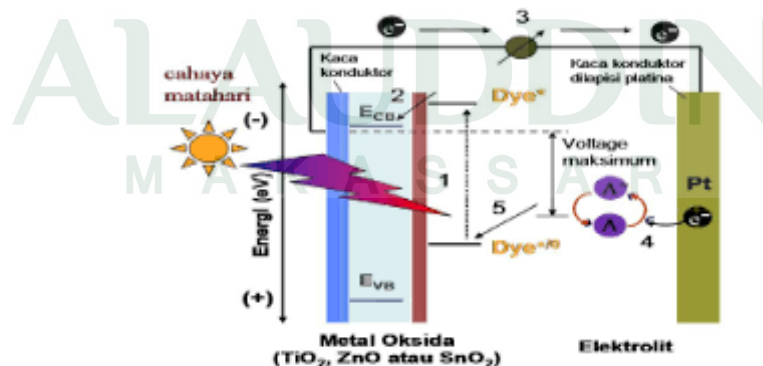
Gambar 2. 3 Prinsip DSSC (Prasada, dkk., 2015: 52)
