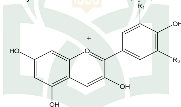
Gambar 2. 4 Struktur Antosianin
