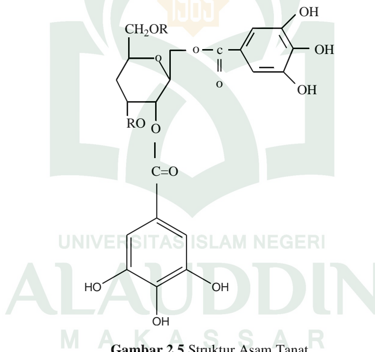
Gambar 2.5 Struktur Asam Tanat
