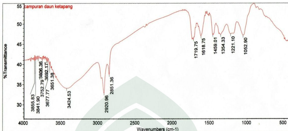
Gambar 4.7 Hasil Serapan IR Ekstrak Daun Ketapang Campuran
