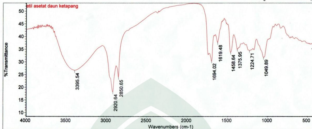
Gambar 4.5 Hasil Serapan IR Ekstrak Daun Ketapang Etil Asetat
