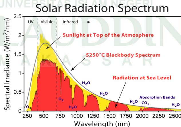
Gambar 2. 1 Spektrum Radiasi Matahari Untuk Cahaya Langsung ke Bumi (Rhodes, 2010: 44)
