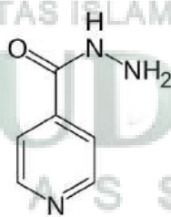
Isoniazid
