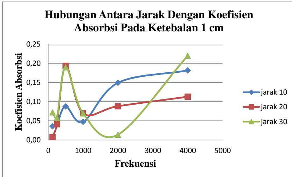
Grafik 4.4 : Pengaruh Jarak SLM Terhadap Koefisien Absorpsi dengan sampel cacahan halus pada ketebalan 1 cm
