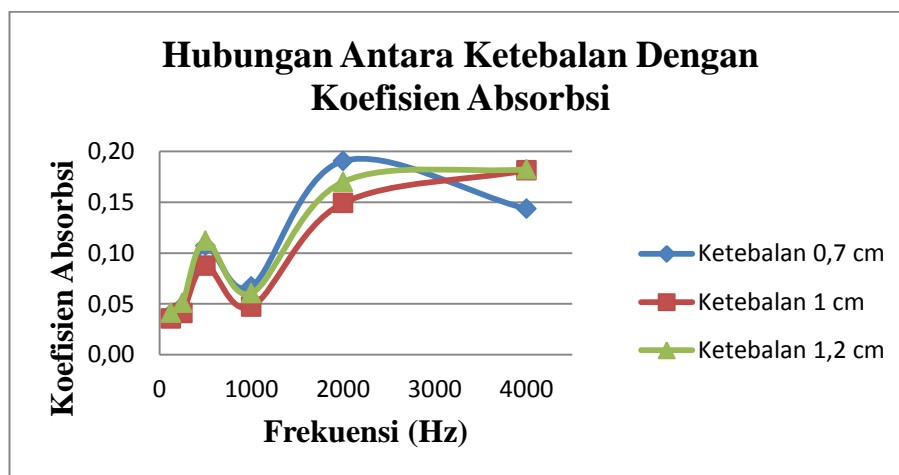
Grafik 4.1: Hubungan antara ketebalan ( x ) dengan koefisien absorpsi ( \alpha ) pada sampel cacahan kasar.
