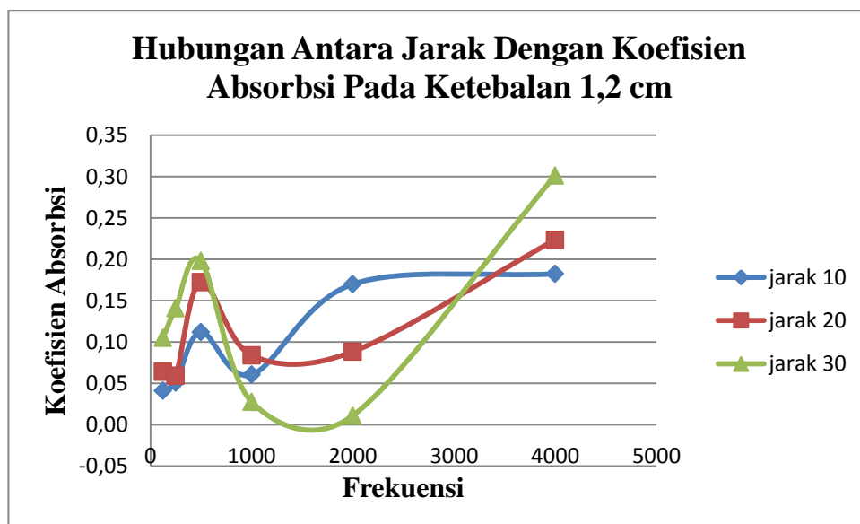
Grafik 4.5: Pengaruh Jarak SLM Terhadap Koefisien Absorpsi dengan sampel cacahan halus pada ketebalan 1,2 cm
