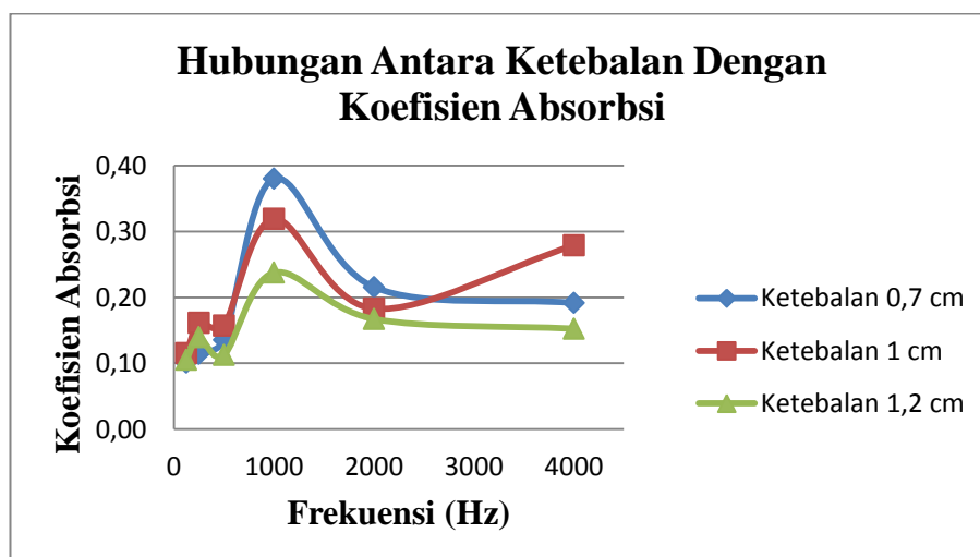
Grafik 4.1: Hubungan antara ketebalan ( x ) dengan koefisien absorpsi ( \alpha ) pada sampel cacahan kasar.
