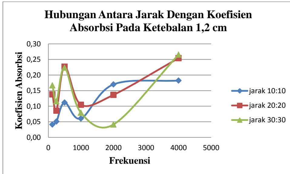
Grafik 4.11: Pengaruh Jarak SLM dan Jarak Sumber Terhadap Koefisien Absorpsi dengan sampel cacahan halus pada ketebalan 1,2 cm.
