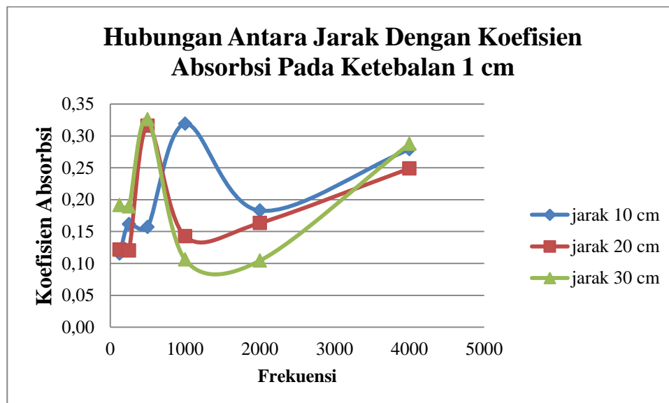
Grafik 4.7 : Pengaruh Jarak SLM Terhadap Koefisien Absorpsi dengan Sampel Cacahan Kasar Pada Ketebalan 1 cm
