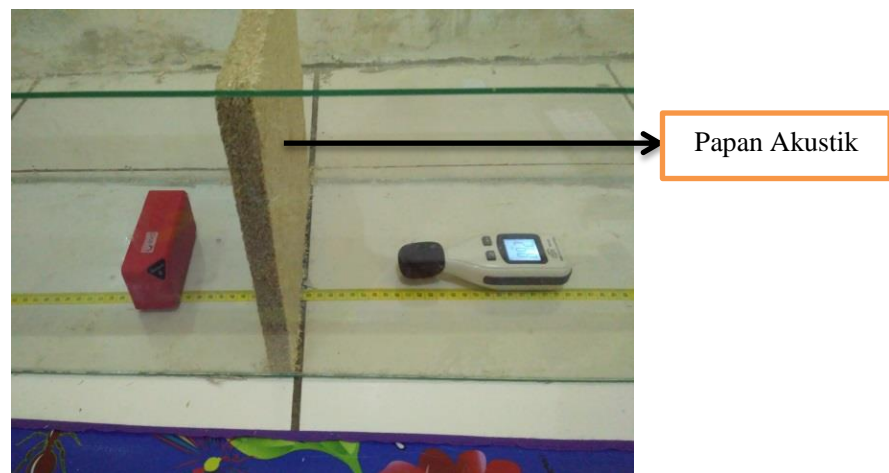
Gambar 4.4: Pengambilan data intensitas akhir ( I )
