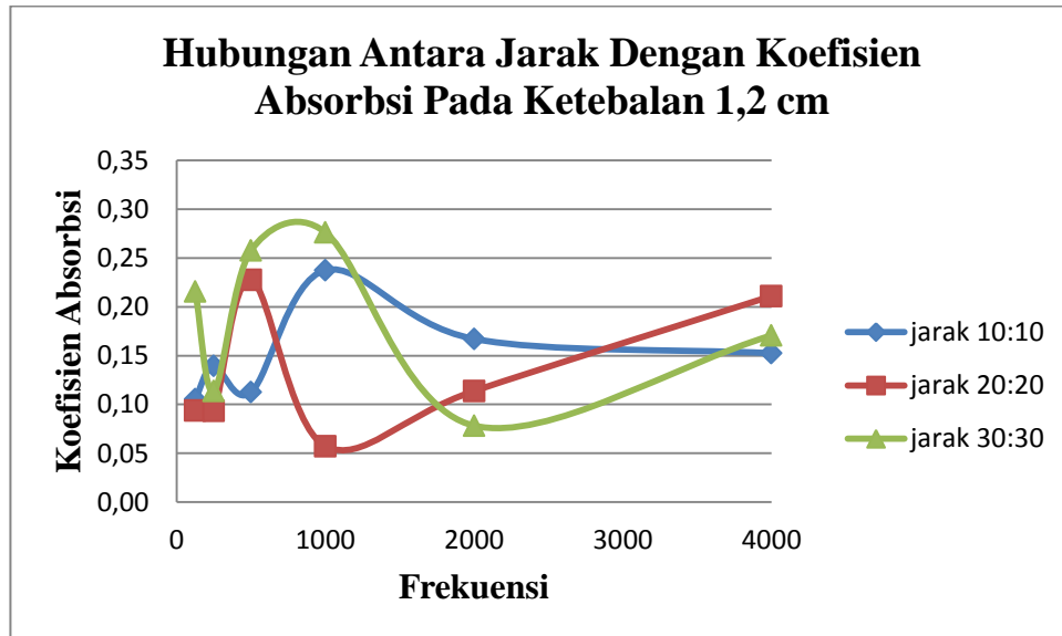
Grafik 4.14: Pengaruh Jarak SLM dan Jarak Sumber Terhadap Koefisien Absorpsi dengan sampel cacahan kasar pada ketebalan 1,2 cm
