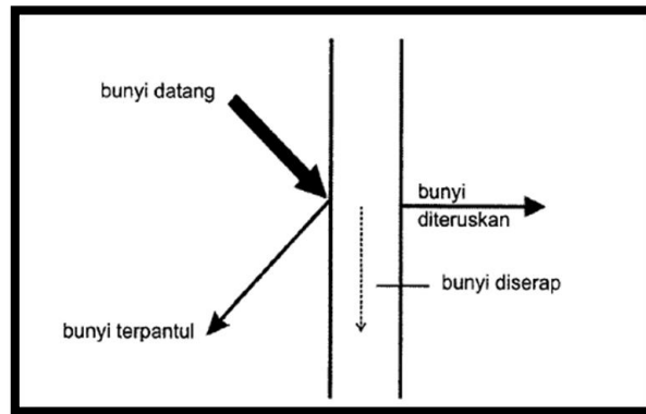
Gambar 2.4 Perambatan gelombang bunyi yang mengenai objek akan mengalami pemantulan dan penyerapan
