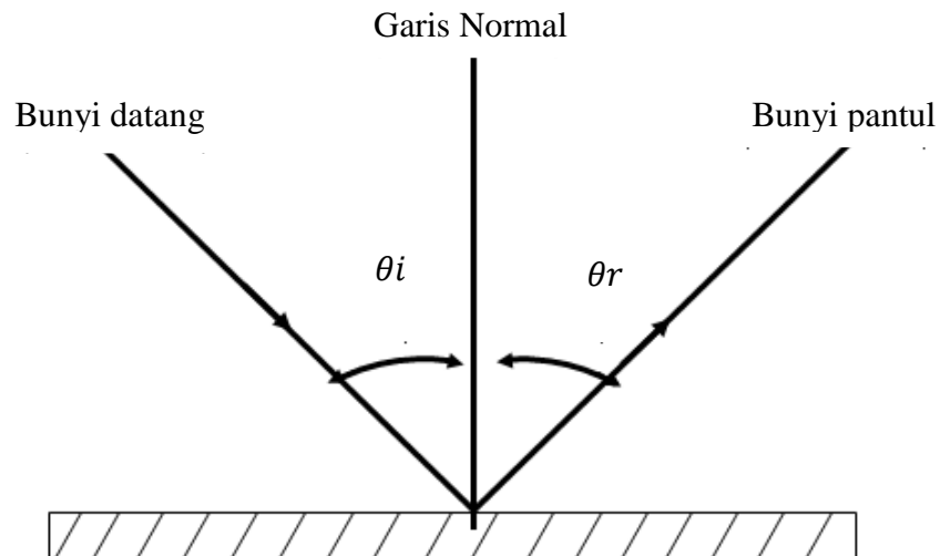
Gambar 2.3 Sifat bunyi yang mengenai bidang (Sumber: J.F Gabriel,2001).
