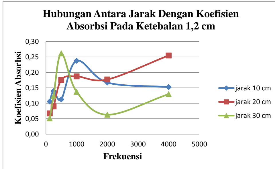
Grafik 4.8 : Pengaruh Jarak SLM Terhadap Koefisien Absorpsi dengan Sampel Cacahan Kasar Pada Ketebalan 1,2 cm
