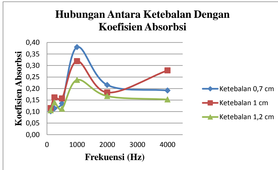
Grafik 4.2: Hubungan antara ketebalan (x) dengan koefisien absorpsi
