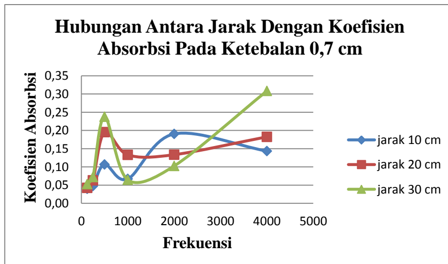
Grafik 4.3: Pengaruh Jarak SLM Terhadap Koefisien Absorpsi dengan sampel cacahan halus pada ketebalan 0,7 cm
