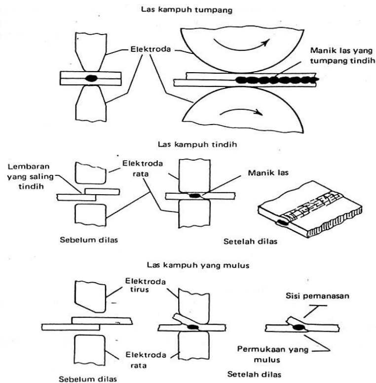
Gambar 2.12. Jenis-jenis las kampuh resistansi listrik.
