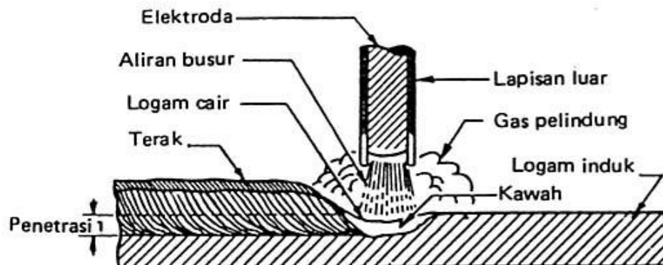
Gambar 2.14. Skema nyala busur.
