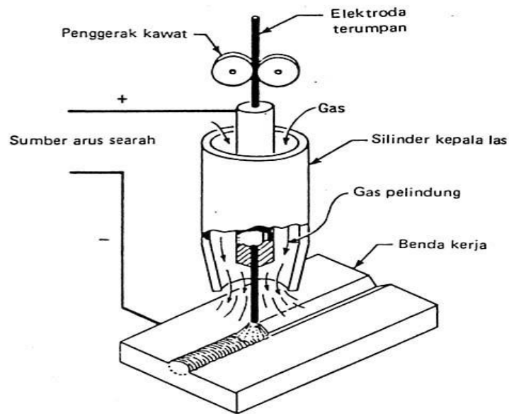
Gambar 2.17. Diagram las busur gas mulia elektroda terumpan.
