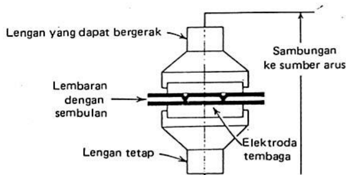
Gambar 2.11 Pengelasan Proyeksi.
