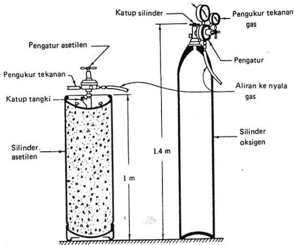
Gambar 2.5 tabung oksigen dan asetilen
