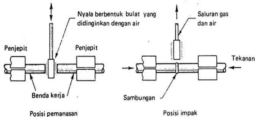
Gambar 2.8 Skema cara pengelasan tumpu dengan gas bertekanan.
