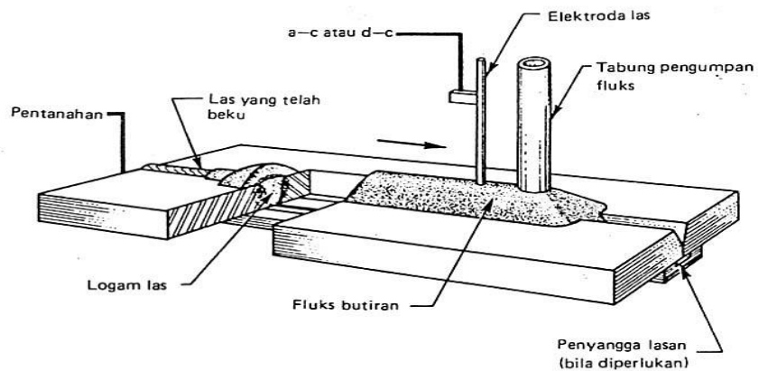
Gambar 2.18. Skema pengelasan busur rendam.
