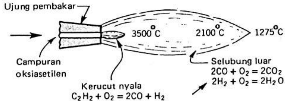
Gambar 2.7. Nyala netral dan suhu yang dicapai pada ujung pembakar.
