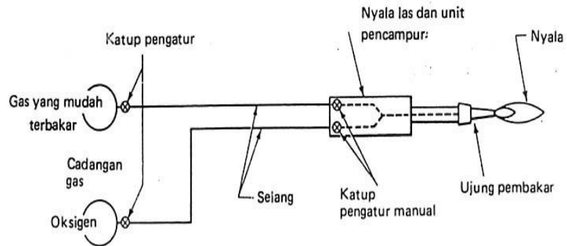
Gambar 2.6 Skema nyala las oksiasetilen dan sambungan gasnya
