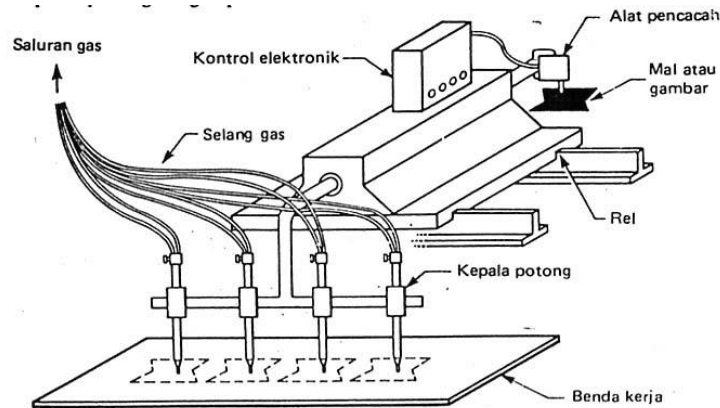
Gambar 2.9. Skema mesin pemotong dengan nyala oksiasetilen.
