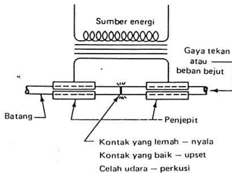
Gambar 2.13 Sketsa pengelasan tumpul.
