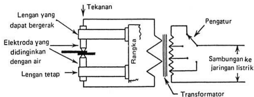
Gambar 2.10. Diagram alat las titik
