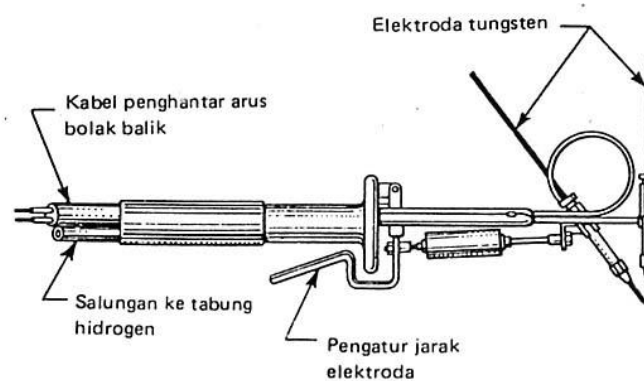
Gambar 2.15. Las busur hidrogen atomik.
