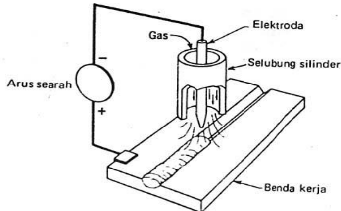
Gambar 2.16. Diagram proses las busur wolfram gas mulia.
