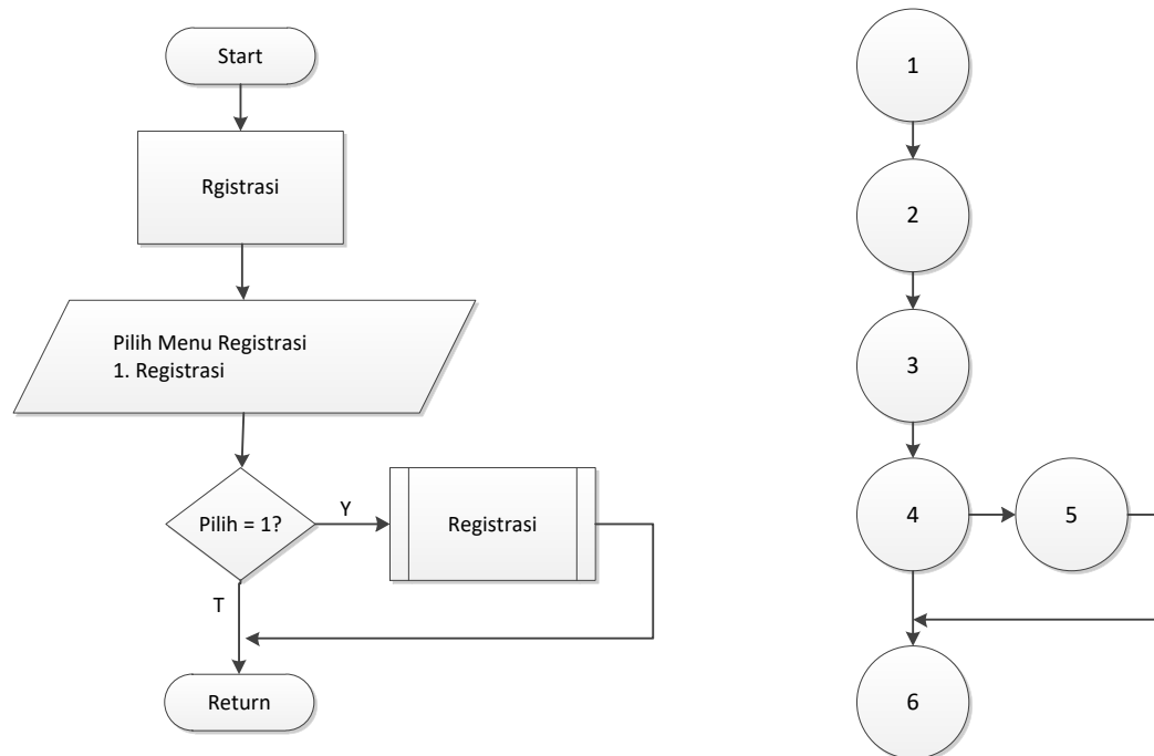
Gambar V.28 Flowchart dan Flowgraph Menu Registrasi
