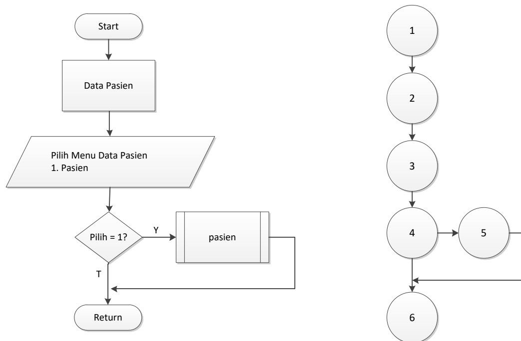
Gambar V.31 Flowchart dan Flowgraph Menu Data Pasien
