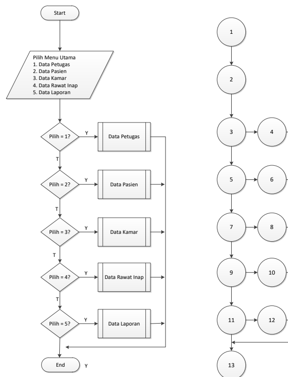
Gambar V.29 Flowchart dan Flowgraph Menu Utama
