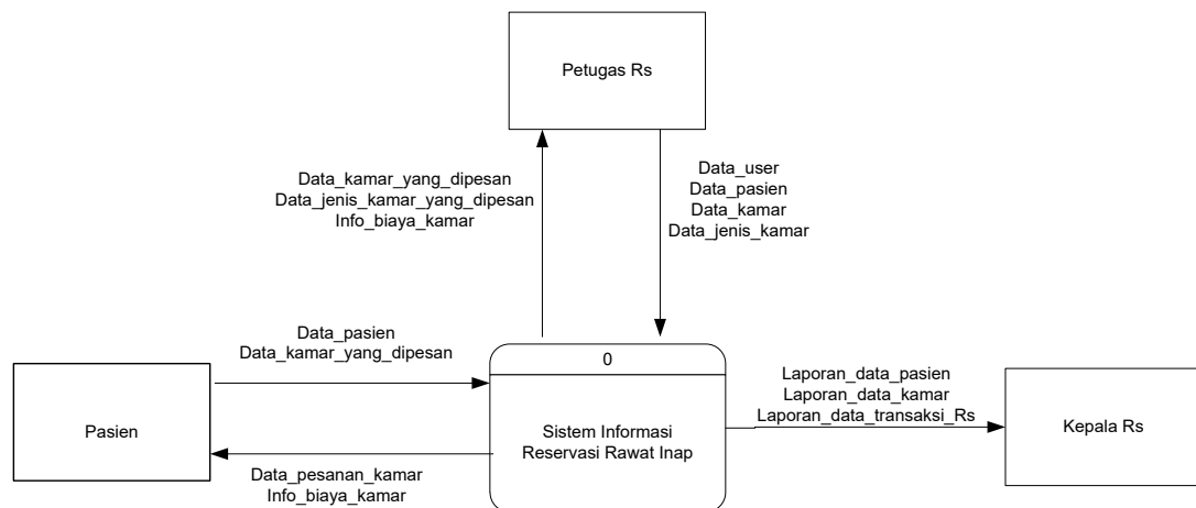
Gambar IV. 3. Diagram Konteks Reservasi Rawat Inap
