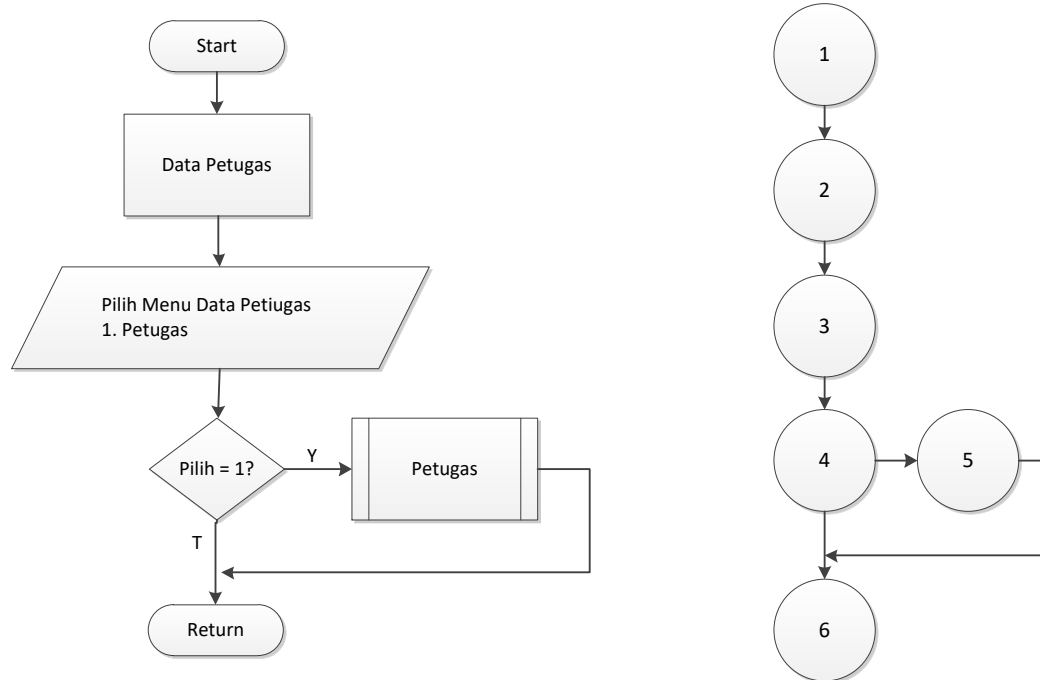
Gambar V.30 Flowchart dan Flowgraph Menu Data Petugas
