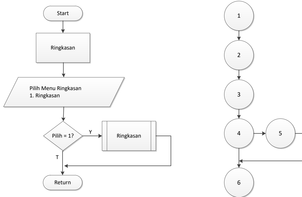
Gambar V.24 Flowchart dan Flowgraph Menu Ringkasan
