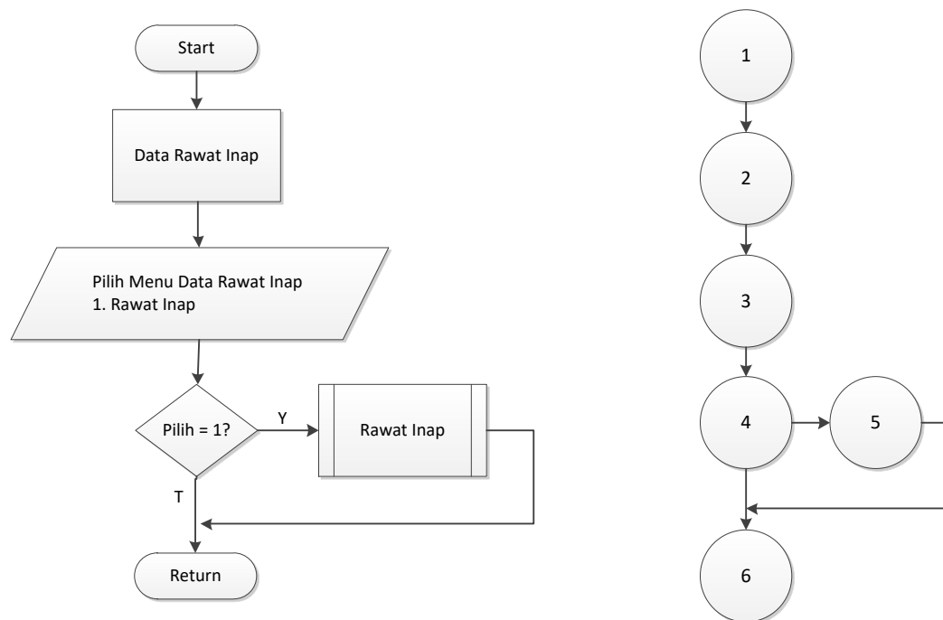
Gambar V.33 Flowchart dan Flowgraph Menu Rawat Inap
