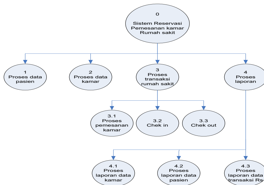
Gambar IV. 4. Diagram Berjenjang
