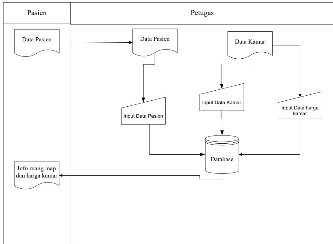
Gambar IV. 2. Bagan Aliran Dokumen Sistem yang Diusulkan
