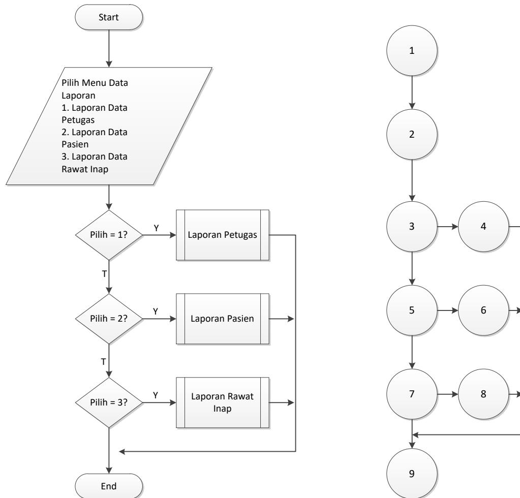
Gambar V.34 Flowchart dan Flowgraph Menu Data Laporan
