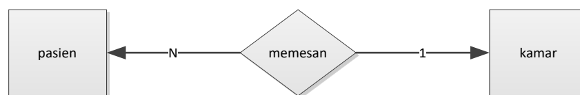
Gambar IV. 8 Diagram ER
