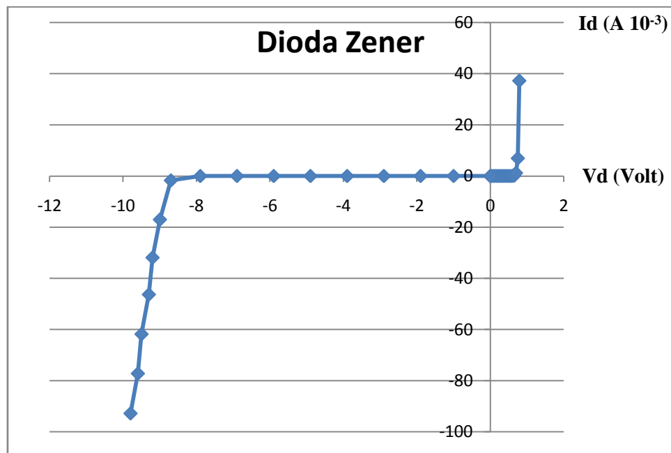
Gambar IV.3 Grafik hubungan antara arus ( I_d ) dan tegangan ( V_d ) pada dioda zener
