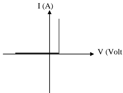
Gambar II.9 Kurva Dioda Pendekatan Kedua
