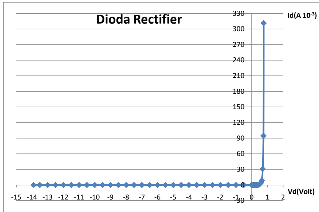
Gambar IV.1 Grafik hubungan antara arus ( I_d ) dan tegangan ( V_d ) pada dioda rectifier.
