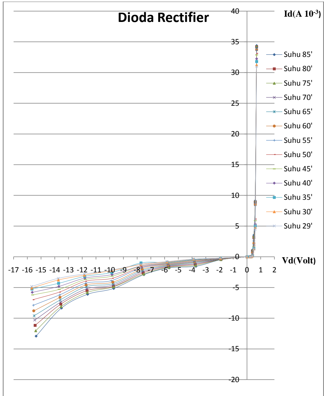
Gambar IV.4. Grafik hubungan antara arus ( I_d ) dan tegangan ( V_d ) pada dioda rectifier setelah dipanaskan
