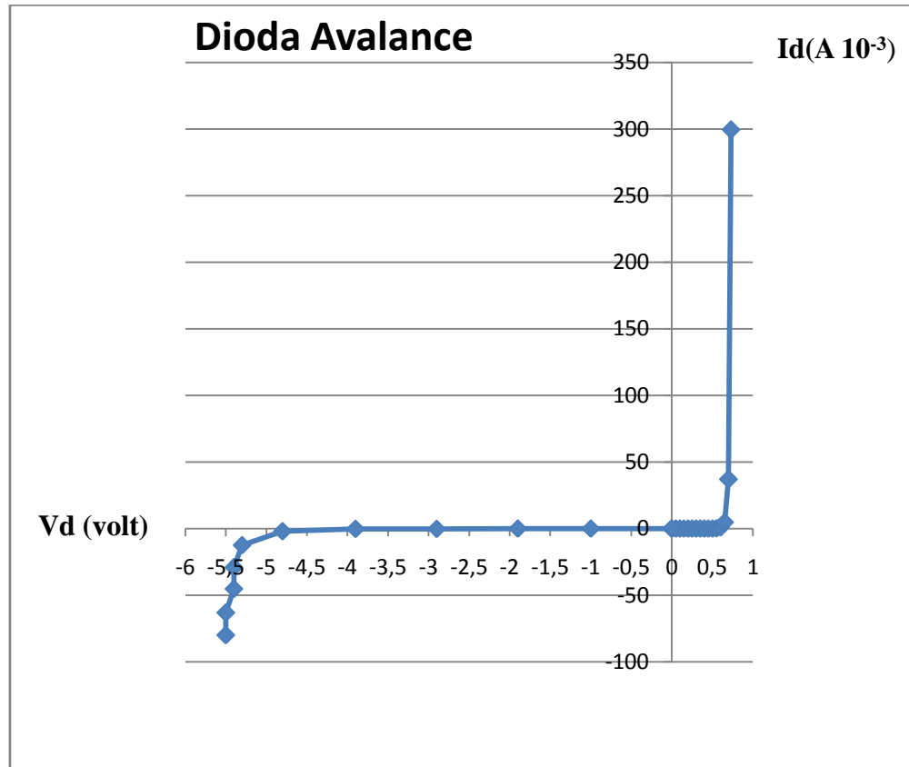
Gambar IV.2 Grafik hubungan antara arus ( I_d ) dan tegangan ( V_d ) pada dioda avalance.
