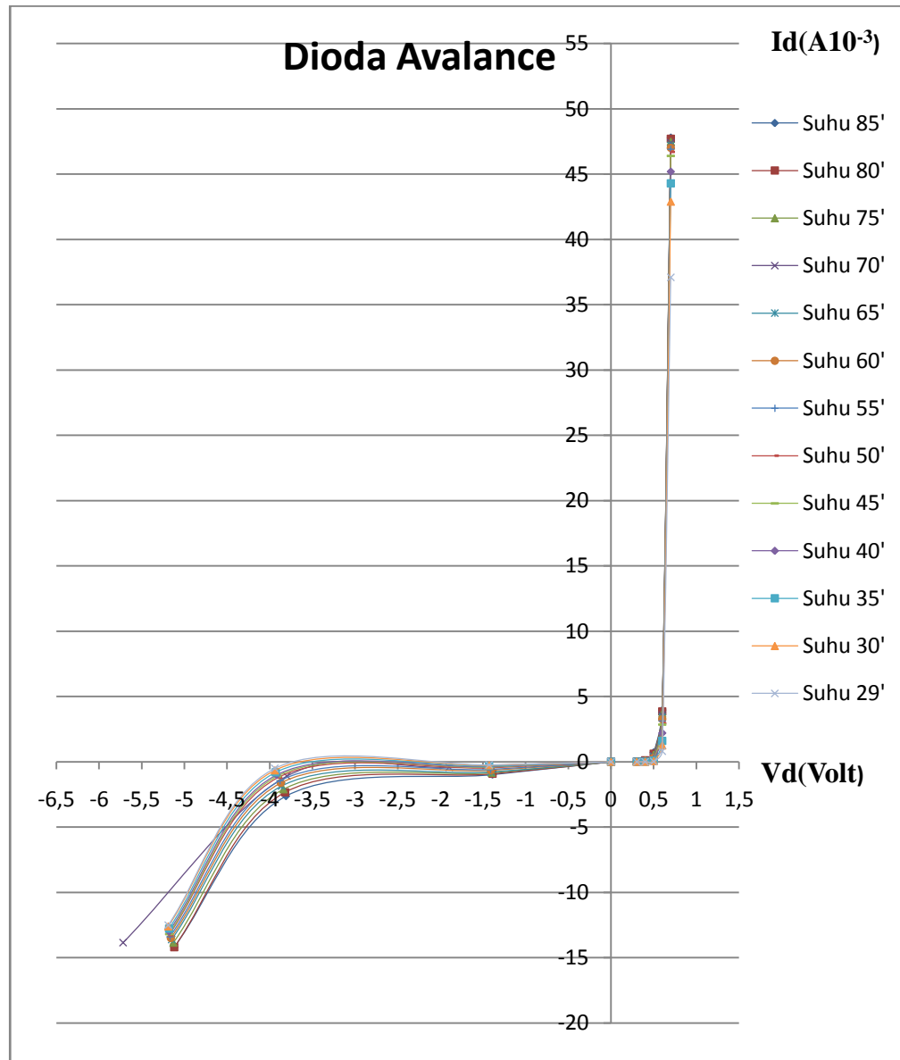
Gambar IV.5. Grafik hubungan antara arus ( I_d ) dan tegangan ( V_d ) pada dioda avalance setelah dipanaskan
