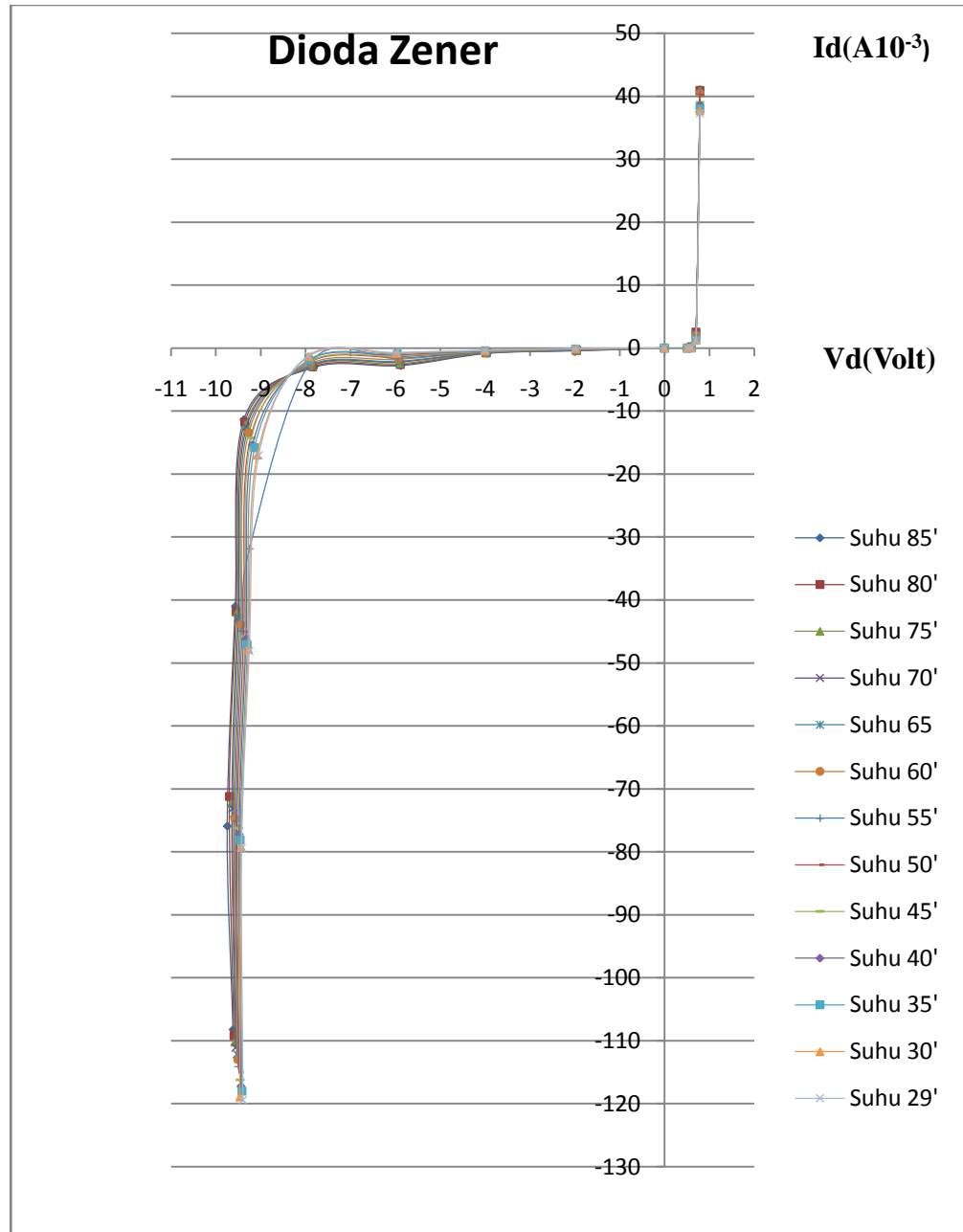
Gambar IV.6. Grafik hubungan antara arus ( I_d ) dan tegangan ( V_d ) pada dioda Zener setelah dipanaskan
