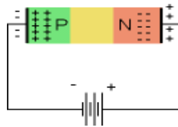
Gambar II.12 Dioda dengan bias negatif
