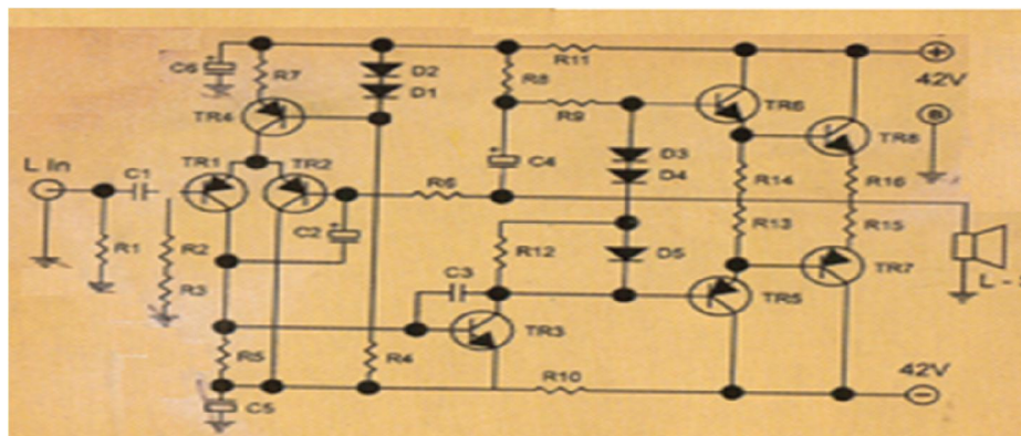
Gambar 3.2. skema rangkaian sebelum dirubah
