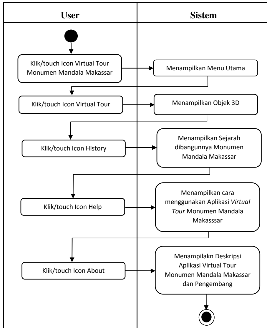
Gambar VI 6 Activity Diagram Menu Utama
