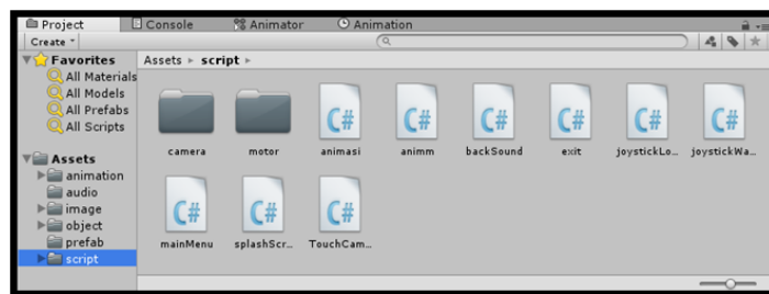
Gambar V.2 Script Aplikasi
