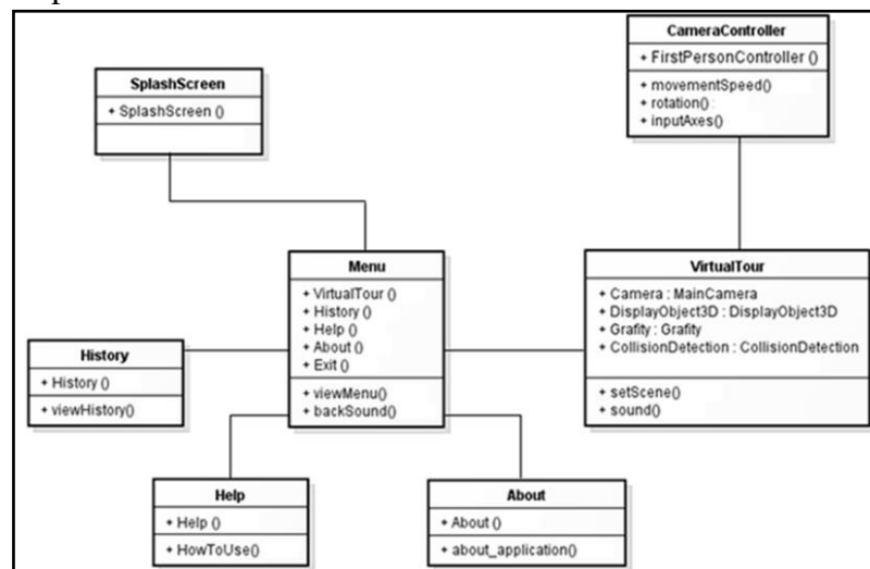
Gambar VI.3 Class Diagram Aplikasi Virtual Tour Monumen Mandala Makassar
