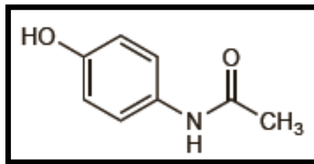
Gambar 1. Rumus struktur parasetamol (Sweetman, 2009; 108)
