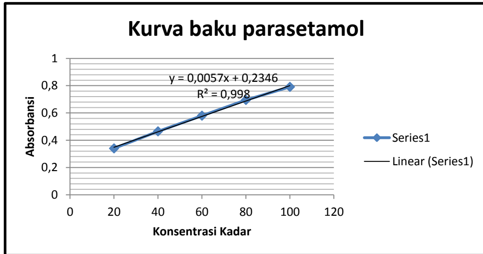
Gambar 6. Kurva baku parasetamol pada panjang gelombang maksimal 289,0 nm
