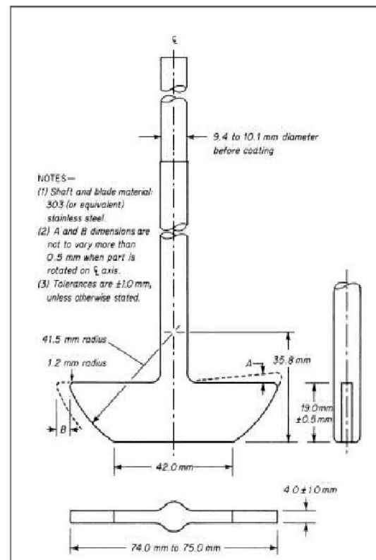
Gambar 3. Pengaduk Bentuk Dayung
