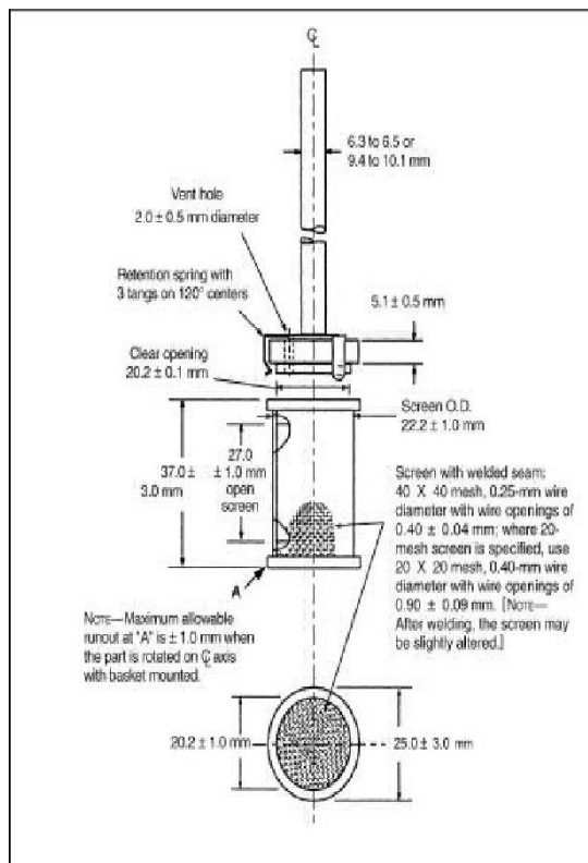
Gambar 2. Pengaduk Bentuk Keranjang
