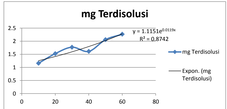
Gambar 8. Kadar Asam Mefenamat Terdisolusi Tiap Satuan Waktu Pada Formula 4
