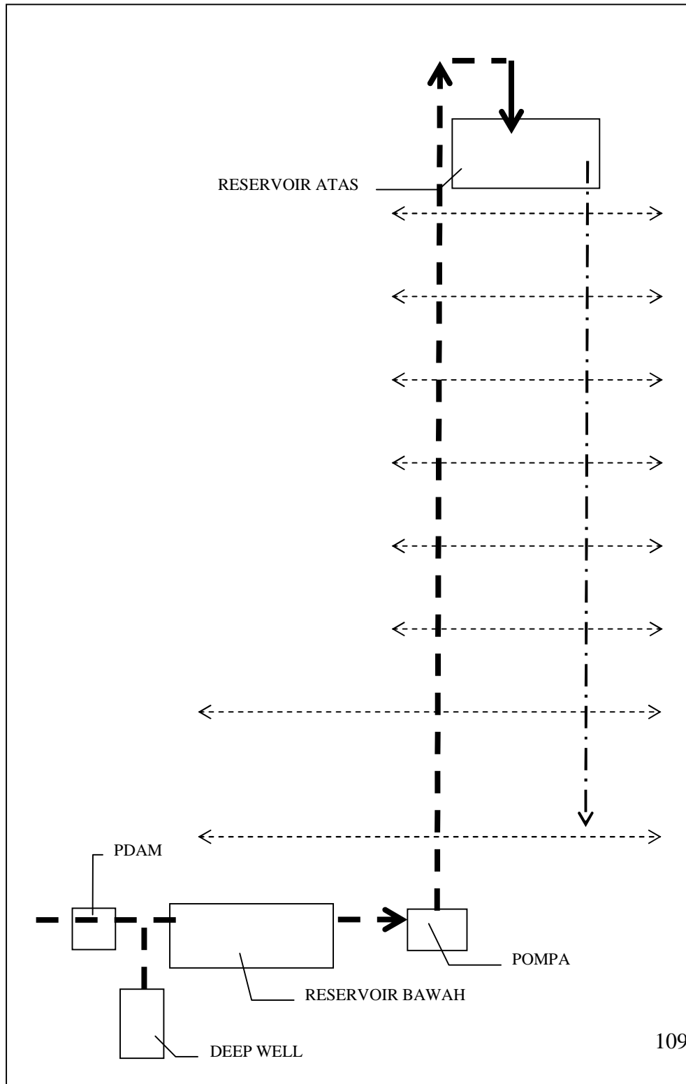
Skema IV.1. Sistem Pengaliran Air Bersih
