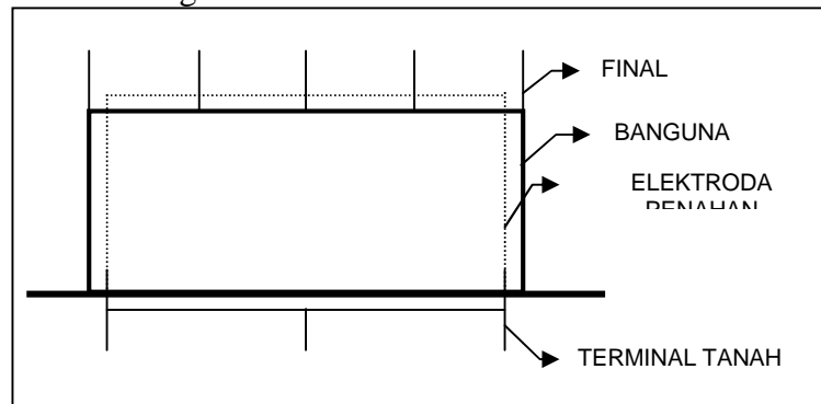
Gambar IV.6. Sistem Sangkar Faraday
