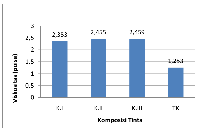
Grafik 4.2 Hubungan nilai viskositas dengan variasi komposisi tinta
