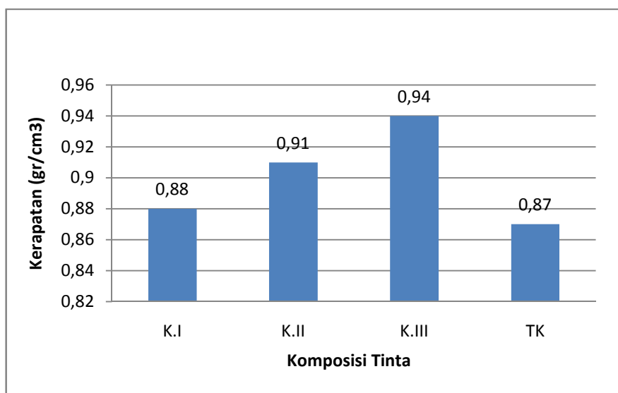
Grafik 4.1 Hubungan nilai kerapatan dengan variasi komposisi tinta
